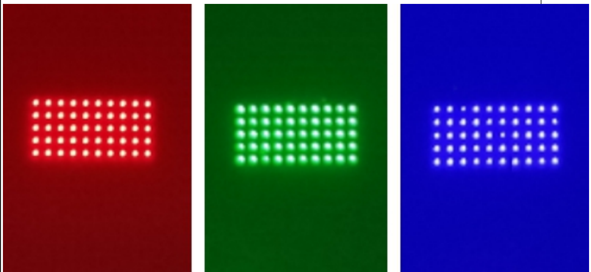
rgb소자 점등 이미지 그림 8. Micro LED칩 실장 후 RGB 소자 점등 이미지
